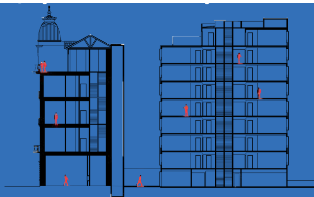
Corte Longitudinal
