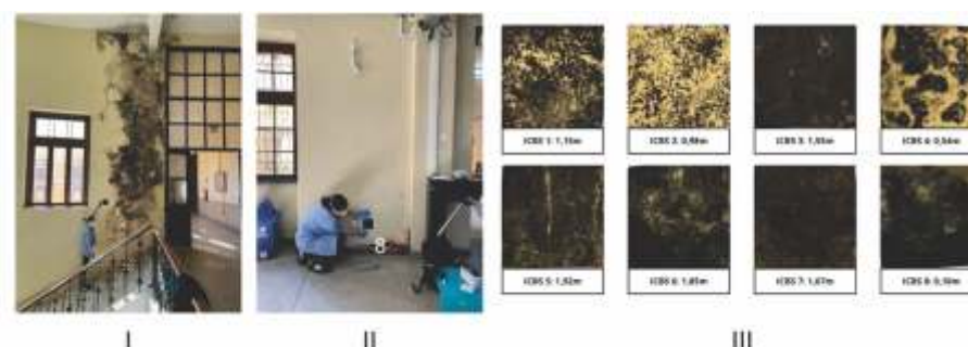
Figura 3: Identificação dos pontos de coleta: (I) pontos de coleta no terceiro pavimento, (II) ponto de coleta no pavimento térreo; (III) pontos de coleta ampliados e respectivas alturas em relação ao piso. Fonte: os autores.
