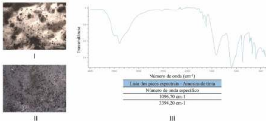
Figura 6: Amostra de tinta (I) e prospecção (II) vistas em lupa estereoscópica; resultado FTIR (III). Fonte: os autores.
