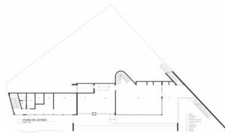
Figura 4: Redesenhos do projeto arquitetônico. Fonte: Redesenhos no Revit produzidos por Antônio Lucas Souza. 2025.
