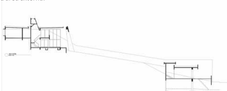
Figura 2: Implantação dos volumes no terreno. Fonte: Redesenhos no Revit produzidos por Antônio Lucas Souza. 2025.
