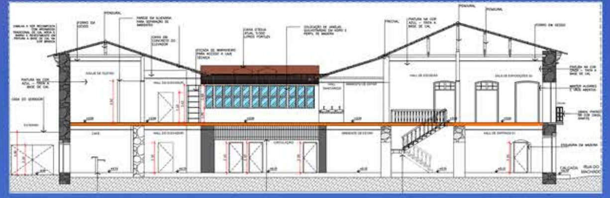
CORTE BB'
