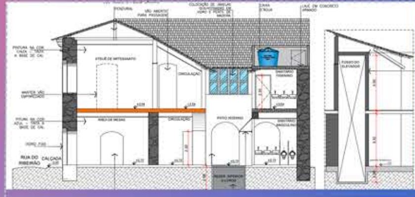
CORTE AA'
